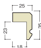
見切り形状
