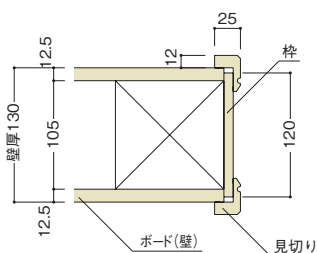
壁厚130mmの場合の納まり例
