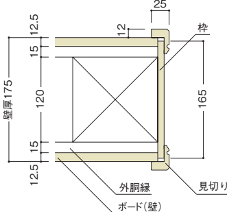
壁厚175mmの場合の納まり例
